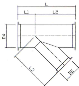
45°Y管
