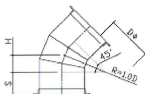
45°ベンド(1R)
