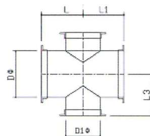
クロス管
